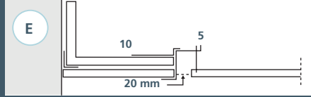
Reunakaista ja Trap-levyn kannatus konsolilla ja reunaprofiililla
