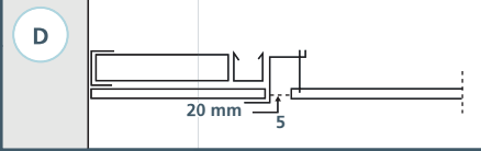
Kiinteän reunakaistan ja Trap-levyn liitos reunaprofiililla
